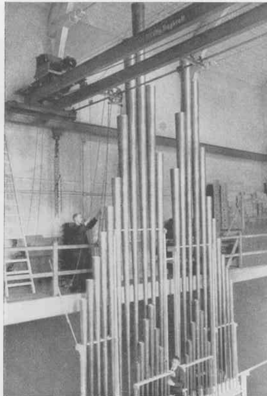
AUFBAU EINER CONTRAPOSAUNE 32'
